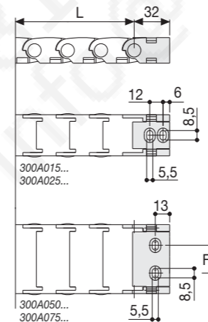
Рис. А Цепь фиксируется по внешнему/внутреннему радиусу (Рис. А)
