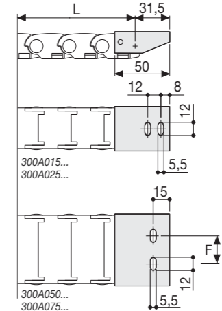
Рис.Б Цепь фиксируется по внешнему радиусу (Рис. Б)
