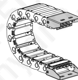
Рис.Б Цепь фиксируется по внешнему радиусу (Рис. Б)
